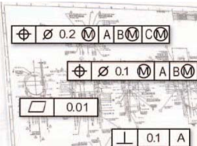
Prüfmerkmale im CAD-Modell
