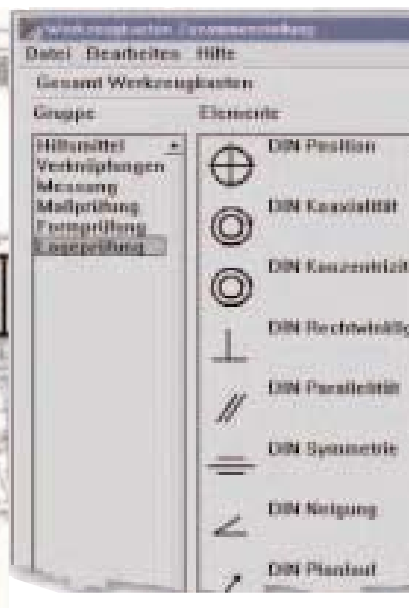
Zusammenstellung des Messprogramms durch Anklicken der Elemente.
