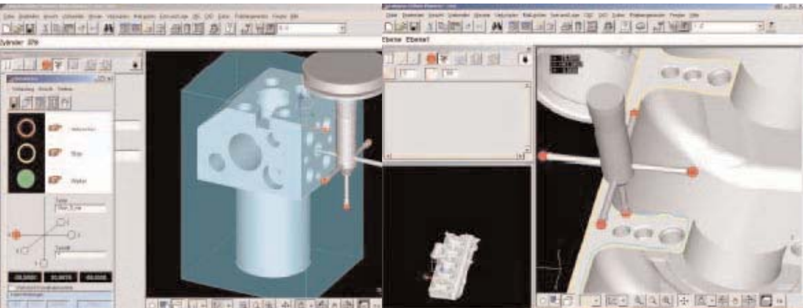
Calypso generiert automatisch die Messbläufe
